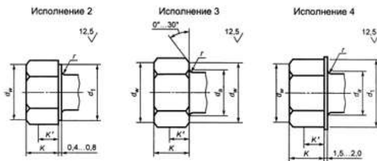
Рисунок А.1 — Конструктивное исполнение тела болта 2
